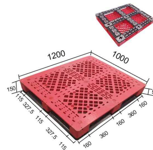
Grid "田" font type 网格田字型 1210-150
