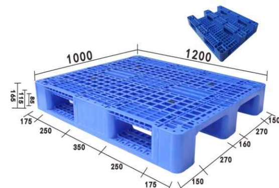
Grid "川" type 网格川字型 1210-165
