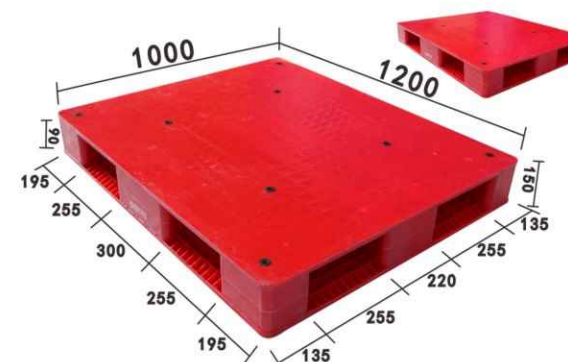
Flat double side type 平板双面型 1210-150
