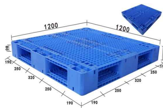
Grid double side type 网格双面型 1212-150
