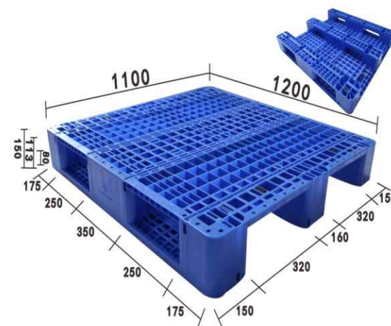
Grid "川" type 网格川字型 1211-150
