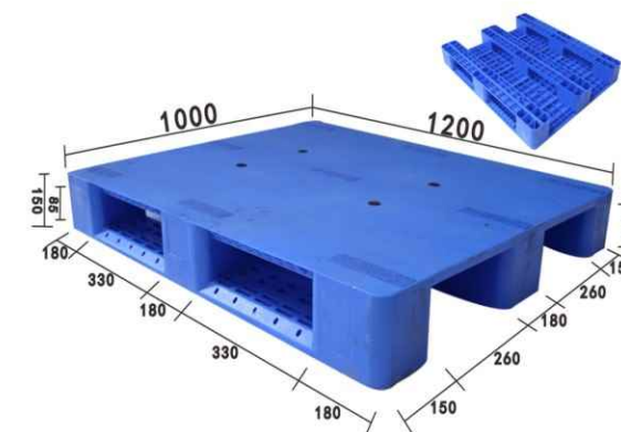
Flat "川" type 平板川字型 1210-150
