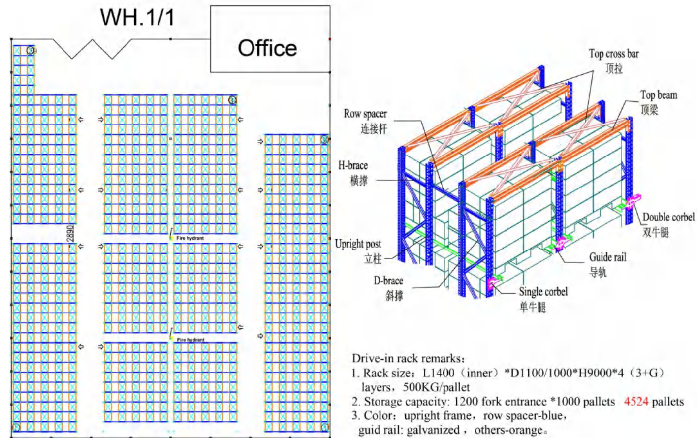
Drive-in rack layout diagram & structure diagram 驶入式货架布局图 & 结构图
