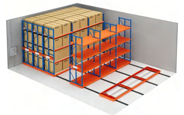
Mobile rack 3D view 移动货架3D效果图
